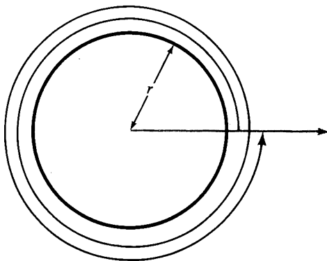
Figura 3.2.1 La longitud de arco de un círculo recorrido dos veces es 4\pi r .
